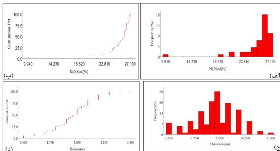
شکل ۳: نمودار الف) هیستوگرام و ب) فراوانی تجمعی داده‌های عیارسنجی، ج) هیستوگرام و د) فراوانی تجمعی داده‌های ضخامت ماده معدنی سولفات سدیم محدوده کویر میقان اراک.
