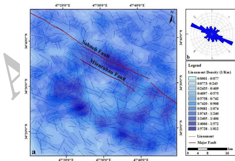
شکل ۳: (a) نقشه تراکم خطواره‌های منطقه مورد مطالعه و (b) دیاگرام گل‌سرخ مربوط به این خطواره‌ها روند غالب N45W تا N65W را نشان می‌دهد. موقعیت دقیق منطقه مورد مطالعه در شکل ۱ مشخص شده است.
