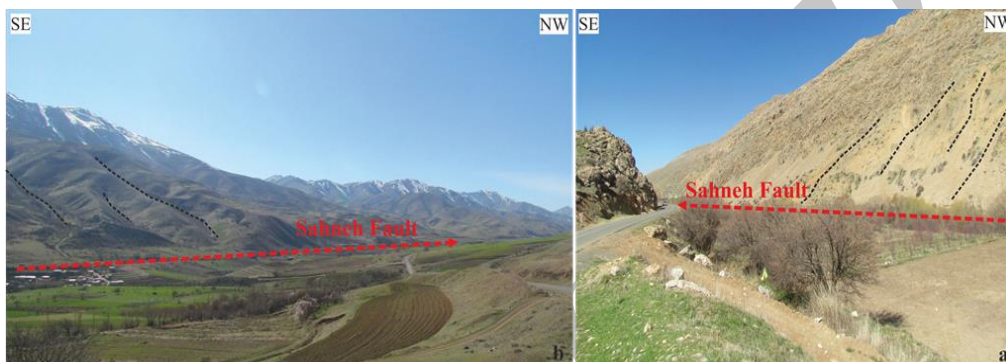
شکل ۹: (a) دره گسلی محل عبور قطعه میانی گسل صحنه و (b) دره گسلی محل عبور قطعه شمال‌باختری گسل صحنه. موقعیت دقیق دره‌های گسلی در شکل ۱ مشخص شده است.
