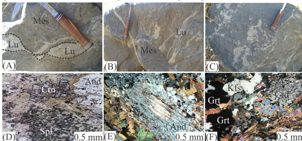
شکل ۵: (A) میگماتیت‌های استروماتیک، (B) میگماتیت‌های شیلرن: از نوارهای تیره و روشن تشکیل شده که نوارها نامنظم بوده و انتهای باریک و مخروطی شکل دارند. (C) میگماتیت‌های لخته‌ای: لوکوسوم به صورت لخته و تکه‌های پراکنده داخل مزوسوم قرار دارد، (D) کانی‌های اسپینل و کروندم در اطراف بلور آندالوزیت در بخش مزوسوم میگماتیت-ها، (E) تبدیل آندالوزیت به سیلیمانیت از حاشیه داخلی، (F) گارنت همراه با مجموعه کانی‌های کوردیریت، بیوتیت، فلدسپار پتاسیم.
