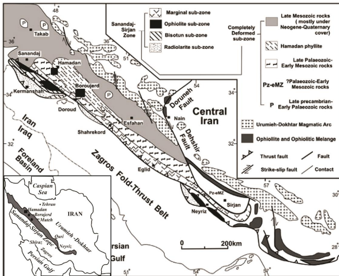
شکل ۱: موقعیت مناطق مورد مطالعه در نقشه زمین‌شناسی ایران و موقعیت تکتونیک زون‌ها در غرب ایران (مجل و همکاران، ۲۰۰۳) موقعیت مناطق مورد مطالعه با علامت مربع نشان داده شده است.
