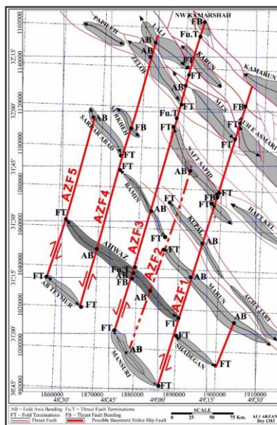
شکل ۹: سیستم گسلی موجود در افق آسماری ناحیه دزفول شمالی (براساس داده‌های لرزه‌ای) (ارزانی و حیدری، ۱۳۸۷).
