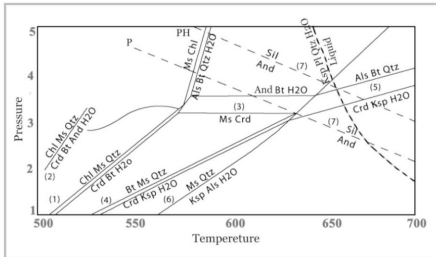
شکل ۶: مدل سیستم پلیتی KFMASH شامل کوردیریت (Crd)، آلومینوسیلیکات‌ها (And, Sil)، پتاسیم فلدسپار (Ksp)، بیوتیت (Bt)، مسکویت (Ms)، کلریت (Chl)، کوارتز (Qtz)، پلاژیوکلاز (Pl)، مکان‌یابی توسط Powell and Holland, (1990) (1990) Spear and Cheney, (1989) (1992) Pattison, 1992، و با علامت PH نقطه سه گانه تعیین شده براساس واکنش And=Sil با علامت P توسط پتیسون، (1992) Pattison، و با علامت PH توسط پاول و هلند (1990) Powell and Holland.
