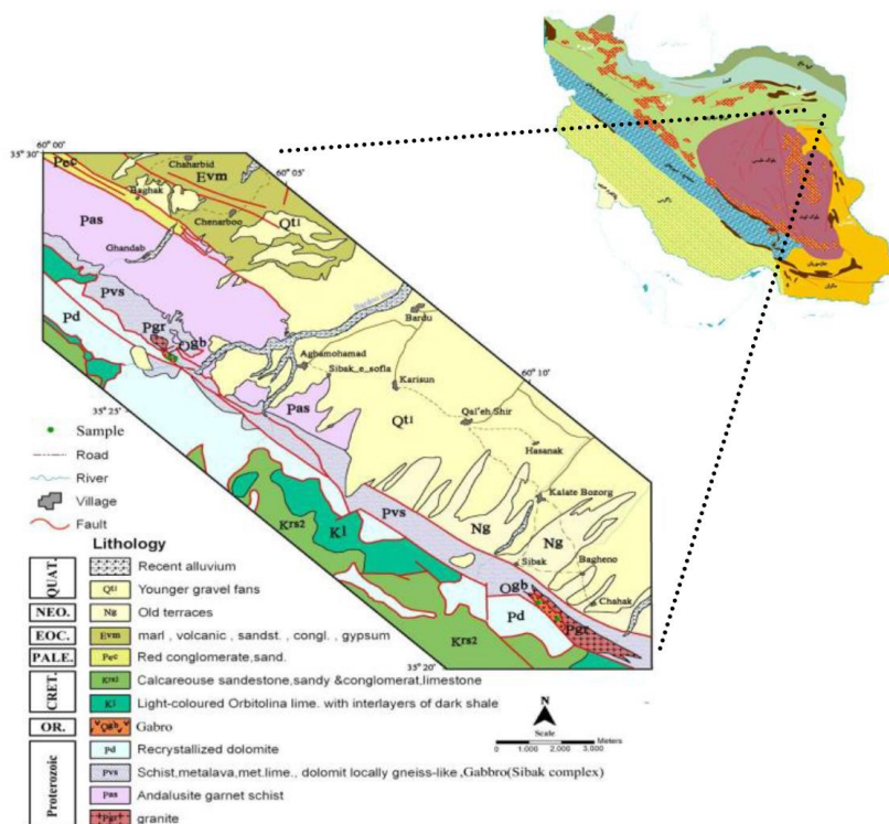
شکل ۱: نقشه زمین‌شناسی منطقه، برگرفته از نقشه با مقیاس ۱/۱۰۰۰۰۰ کاریزنو (۱۹۷۹).
