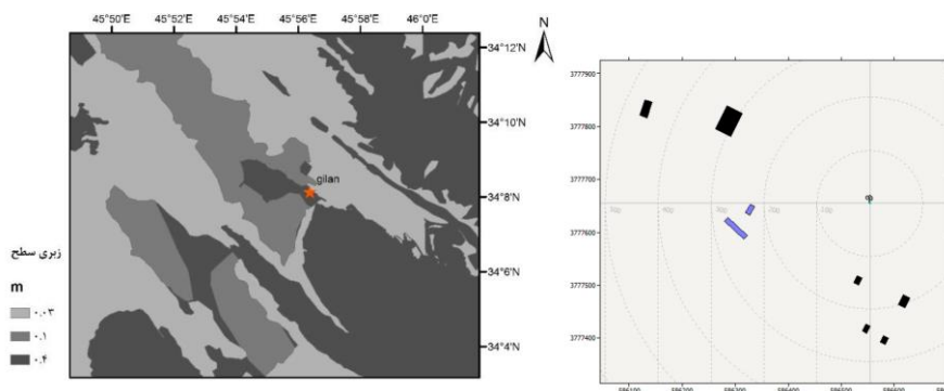
شکل ۱۴: موقعیت موانع شناسایی شده (رنگ مشکی: تخلخل صفر و رنگ آبی تخلخل ۰/۵) و نقشه زبری سطح در محدوده ایستگاه گیلان غرب
