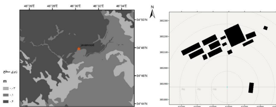
شکل ۱۳: موقعیت موانع شناسایی شده (رنگ مشکی): تخلخل صفر و رنگ آبی تخلخل (۰/۵) و نقشه زبری سطح در محدوده‌ی ایستگاه جوانرود
