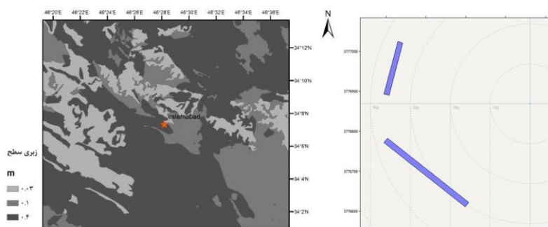
شکل ۸: موقعیت موانع شناسایی شده (رنگ مشکی: تخلخل صفر و رنگ آبی تخلخل 0/5 ) و نقشه زبری سطح در محدوده‌ی ایستگاه اسلام‌آباد غرب
