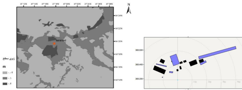
شکل ۹: موقعیت موانع شناسایی شده (رنگ مشکی: تخلخل صفر و رنگ آبی تخلخل ۰/۵) و نقشه زبری سطح در محدوده ایستگاه سرارود
