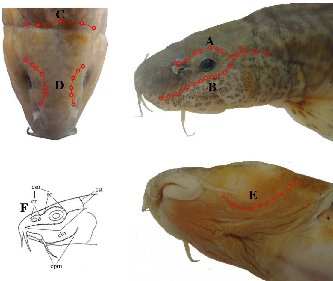
شکل ۱۲. موقعیت قرارگیری کانال‌های حسی سر گونه P. rhadinæa و A: D: B. Commissura supratemporalis: C: Canalis supraorbitalis: E: Canalis infraorbitalis: F: مدل معرفی شده کانال‌های حسی سر جنس Paracobitis برگرفته از Prokofiev (2009).
