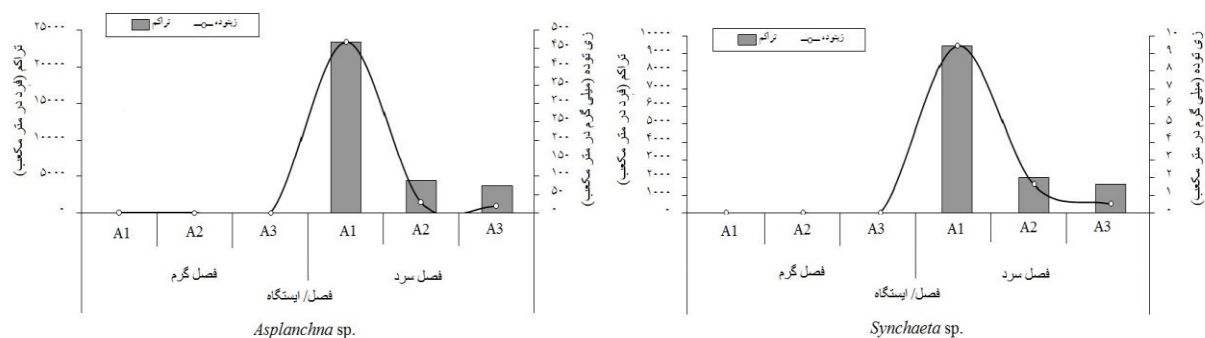
شکل ۳. تراکم و زی توده فصلی و مکانی Synchaeta sp. و Asplanchna sp. از گردان ننان (ایستگاه A 1 عمق ۵-۰ متر)؛ ایستگاه A 2 عمق ۱۰-۰ متر)؛ ایستگاه A 3 عمق ۲۰-۰ متر)؛ ایستگاه A 3 عمق ۲۰-۰ متر)
