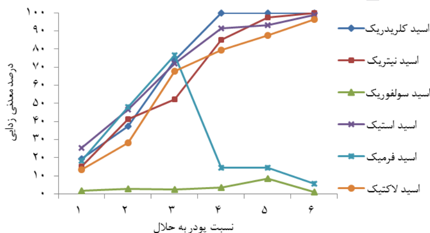
شکل ۲. اثر نسبت پودر به حلال روی حذف ترکیبات معدنی پودر پوسته‌ی خرچنگ P. segnis . نسبت ۱:۵، ۱:۲، نسبت ۱:۱۰، ۳:۱ نسبت ۱:۱۵، ۴:۱، نسبت ۱:۲۰، ۵:۱ نسبت ۱:۲۵ و ۶:۱، نسبت ۱:۳۰
