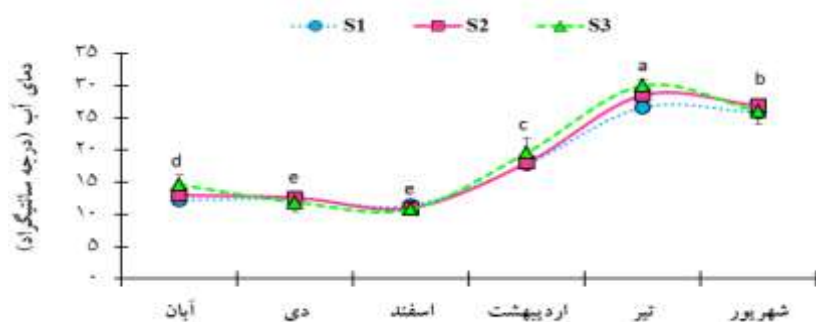
شکل ۲. مقایسه میانگین (± انحراف معیار) دمای آب برحسب ایستگاه‌ها و ماه‌های مختلف نمونه‌برداری در مصب سردآبرود چالوس (S1: اکوسیستم رودخانه، S2: اکوسیستم مصب و S3: اکوسیستم دریا). حروف نامتشابه بیانگر اختلاف معنی‌دار در بین میانگین‌هاست (P<0.05).
