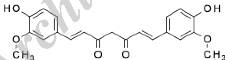
شکل ۱) ساختار کورکومین
