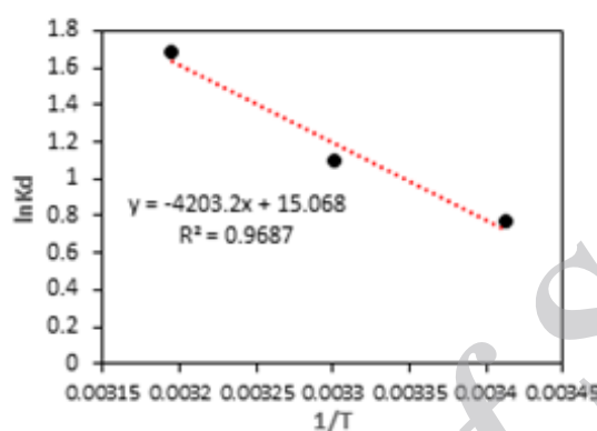
شکل ۴- نمودار وانتروف برای پیش بینی پارامترهای ترمودینامیکی جذب \text{Pb(II)} بر \text{Fe}_3\text{O}_4\text{-NH}_2
