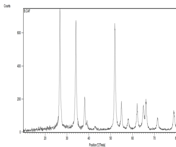
شکل (۳). الگوی پراش پرتو ایکس نانو اکسیدتهپیه شده \text{SnO}_2
