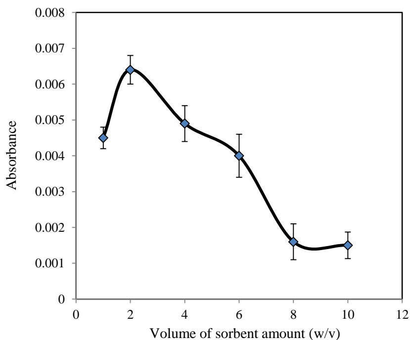
شکل ۴: بهینه‌سازی نوع ماده جاذب. ۰/۵ mL متانول و آمونیوم دی‌تیوکاربامات 1 \mu\text{g/mL} در pH برابر با ۴
