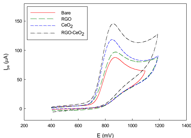
شکل ۳- ولتاموگرام اکسایش سولفادیازین روی الکترودهای خمیر کربن ساده، خمیر کربن حاوی سریم اکسید، گرافن اکسید کاهش یافته و نانوکامپوزیت
