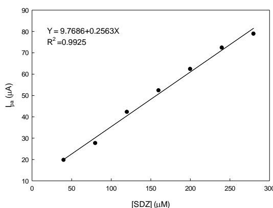
شکل ۹- نمودار کالیبراسیون نمونه حقیقی SDZ (محلول‌ها ۴۰، ۸۰، ۱۲۰، ۱۶۰، ۲۰۰، ۲۴۰ و ۲۸۰ میکرومولار، بافر فسفات pH=۷/۴ و سرعت رویش ۰/۱ ولت بر ثانیه).
