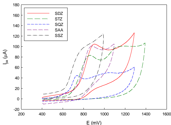
شکل ۲- ولتاموگرام اکسایش مشتقات سولفونامیدی روی الکتروود خمیر کربن اصلاح شده با نانو ذرات CeO_2 حاوی غلظت ۱ میلی مولار نمونه در محلول بافر فسفاتی (pH=۷/۴) با سرعت رویش ۰/۱ ولت بر ثانیه.
