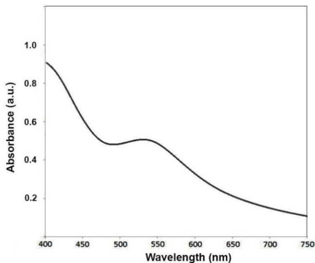
شکل ۱۲- طیف جذبی نانوذرات \text{Au}/\text{Fe}_3\text{O}_4
