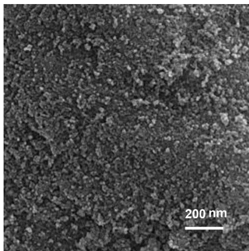
شکل ۳- تصویر میکروسکوپ الکترونی روبشی نانوذرات Au/Fe_3O_4
