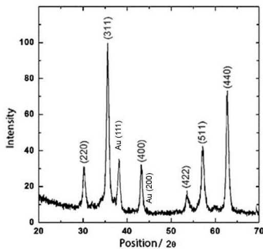
شکل ۲- الگوی پراش پرتو ایکس نمونه سنتز شده Au/Fe_3O_4
