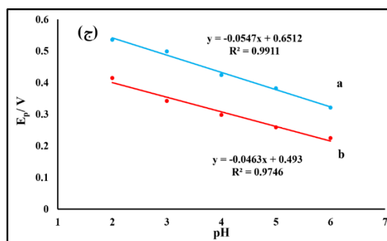
شکل ۴-الف) ولتاموگرام‌های چرخه‌ای کورکومین 10^{-4} M در محلول بافر فسفات 0.1 M حاوی سدیم کلراید 1 M در pHهای متفاوت: (a) ۲، (b) ۳، (c) ۴، (d) ۵، (e) ۶، (f) ۷ و (g) ۸ در سطح CPE در سرعت روبش 100 mV/s در چرخه‌ی دوم. (ب) نمودار جریان دماغه‌های اکسایشی (a) و کاهش‌ی (b) بر حسب pH. (ج) نمودار پتانسیل دماغه‌های اکسایشی (a) و کاهش‌ی (b) بر حسب pH.
