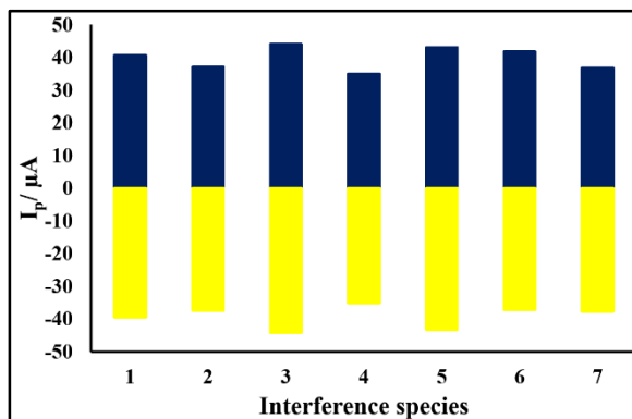
شکل ۶- اثر گونه‌های مزاحم بر جریان دماغه‌های اکسایشی و کاهش کورکومین 10^{-6} M در محلول بافر فسفات 0.1 M ( \text{pH}=3 ) حاوی سدیم کلراید 1 M در سطح CPE در حضور (۱) کورکومین، (۲) کورکومین و \text{K}^+ ، (۳) کورکومین و \text{Cu}^{2+} ، (۴) کورکومین و \text{Ni}^{2+} ، (۵) کورکومین و گلوکز، (۶) کورکومین و ساکاروز و (۷) کورکومین و مخلوطی از هر پنج ترکیب. غلظت هر یک از ترکیبات مزاحم 10^{-2} M است.
