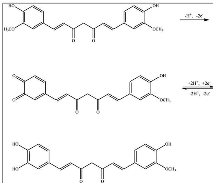
شما تیک ۱- واکنش پیشنهادی فرآیند اکسایش و کاهش کورکومین در سطح CPE [۲۸]
