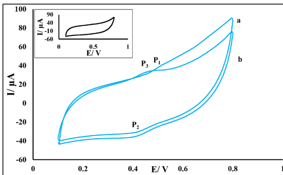
شکل ۲- ولتاموگرام‌های چرخه‌ای کورکومین 10^{-4} \text{ M} در محلول بافر فسفات 0.1 \text{ M} ( \text{pH}=3 ) حاوی سدیم کلراید 1 \text{ M} در سطح CPE در سرعت رویش 100 \text{ mV/s} . کادر درون شکل ولتاموگرام چرخه‌ای CPE را در محلول شاهد بافر فسفات 0.1 \text{ M} ( \text{pH}=3 ) حاوی سدیم کلراید 1 \text{ M} در سرعت رویش 100 \text{ mV/s} نشان می‌دهد.
