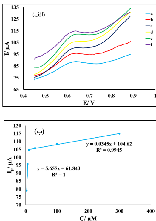
شکل ۵-الف) ولتاموگرام‌های پالس تفاضلی کورکومین با غلظت‌های متفاوت: (a) ۳، (b) ۶، (c) ۱۰، (d) ۳۰، (e) ۱۰۰ و (f) ۳۰۰ \mu\text{M} در محلول بافر فسفات 0.1 \text{ M} (pH=۳) حاوی سدیم کلراید 1 \text{ M} در سطح CPE در سرعت روبش 100 \text{ mV/s} . (ب) نمودار معیارگیری بر مبنای داده‌های قسمت الف.
