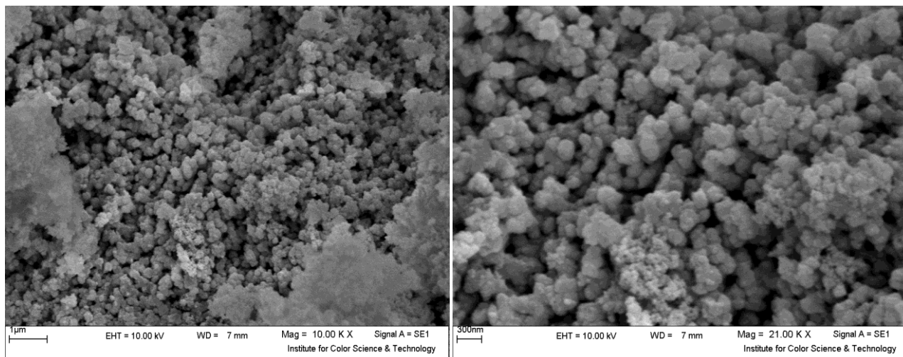
شکل ۱- تصویر SEM نانو ذرات اکسید زیرکونیای غنی شده با کربن فعال در بزرگ‌نمایی‌های مختلف
