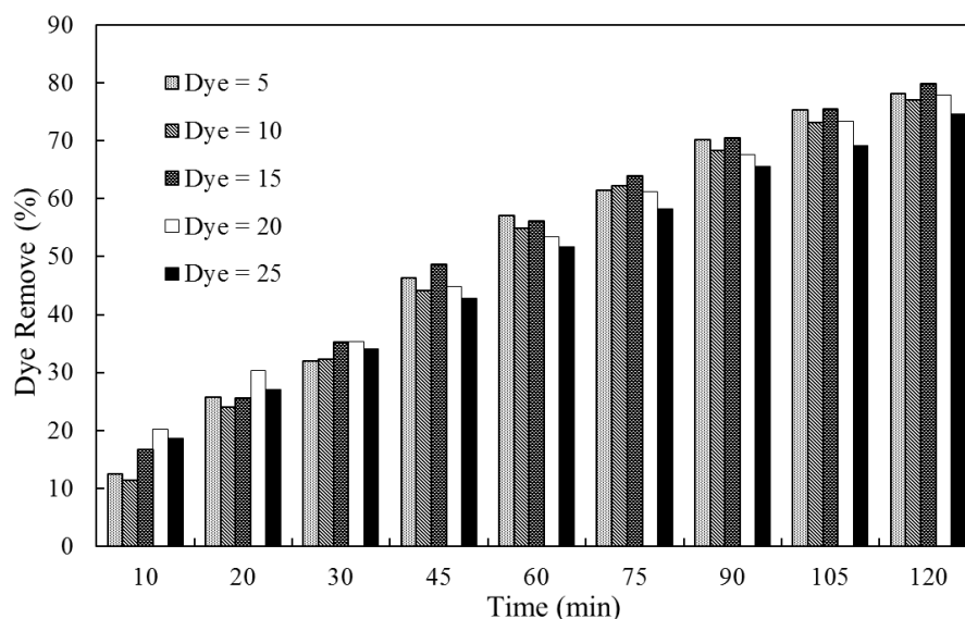
شکل ۳- تأثیر غلظت اولیه رنگ (۵، ۱۰، ۱۵، ۲۰ و ۲۵ میلی‌گرم بر لیتر) بر حذف BR46 در شرایط ثابت (pH=۵، میزان کاتالیزور ۰/۰۶ گرم بر لیتر و توان لامپ ۱۵ وات).
