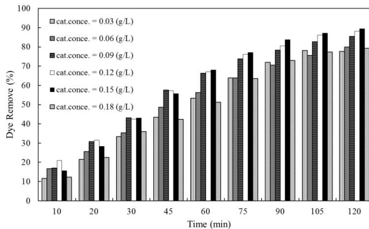
شکل ۵- تاثیر غلظت نانوکاتالیزور ZrO 2 -C (۰/۰۳، ۰/۰۶، ۰/۰۹، ۰/۱۲، ۰/۱۵ و ۰/۱۸ گرم بر لیتر) بر حذف BR46 در شرایط ثابت (pH=۵، غلظت اولیه رنگ ۱۵ میلی گرم بر لیتر و توان لامپ ۱۵ وات).
