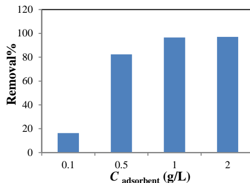
شکل ۶: اثر غلظت کربن فعال بر جذب زرد آلیزارین (دما ۲۵°C، زمان ۴۸ ساعت، غلظت اولیه زرد آلیزارین ۱۰ mg/L).
