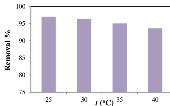
شکل ۵: اثر دما بر جذب زرد آلیزارین توسط کربن فعال ساخته شده از سبوس برنج (غلظت جاذب 1 \text{ g/L} ، زمان ۴۸ ساعت، غلظت اولیه زرد آلیزارین 10 \text{ mg/L} ).
