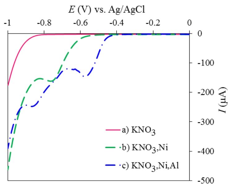
شکل ۱. LSV گرفته شده با روبش پتانسیل از ۰ تا -۱V و سرعت روبش ۱۰ mV.s -1 در محلول (a) KNO 3 ، (b) KNO 3 ,Ni و (c) KNO 3 ,Ni,Al
