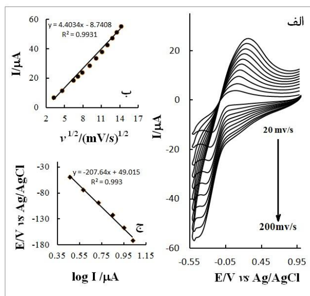
شکل ۴- (الف) ولتامتری چرخه‌ای الکتروکد خمیر گرافن در سرعت روبش‌های مختلف در محلول ۰/۱ مولار بوریک اسید (pH=۳) حاوی ۱ mM اورانیل. سرعت‌های روبش ۲۰، ۴۰، ۶۰، ۸۰، ۱۰۰، ۱۲۰، ۱۴۰، ۱۶۰، ۱۸۰ و ۲۰۰ mV/s، (ب) تغییرات جریان پیک احیای اورانیل با ریشه دوم سرعت اسکن (د) نمودار تافل مربوط به ولتاموگرام در سرعت اسکن ۲۰ mV/s
