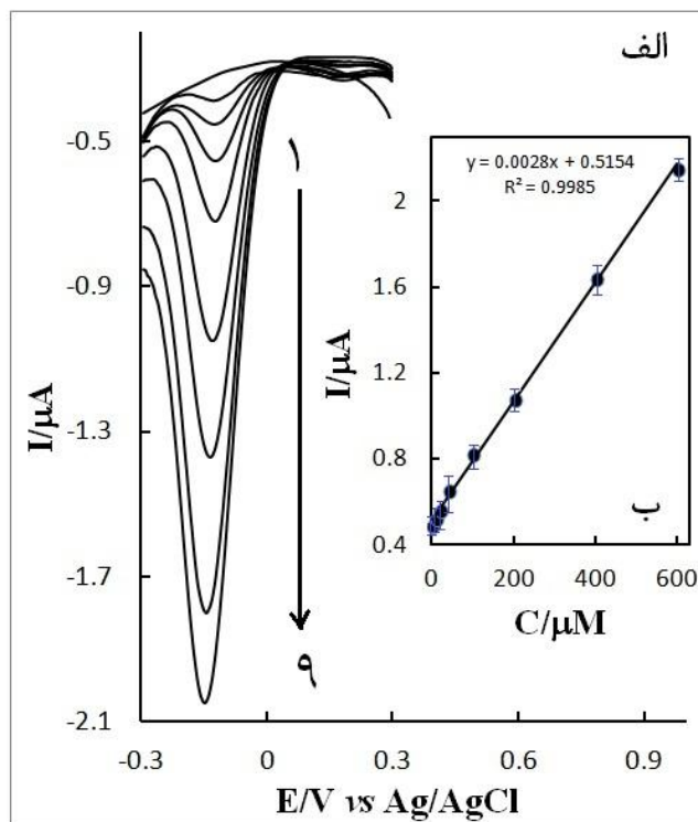
شکل ۵- الف) ولتاموگرامهای پالس تفاضلی محلول زمینه (۱) و محلول‌های (۲ تا ۹) حاوی غلظت‌های ۱، ۲، ۴، ۱۰، ۲۰، ۴۰، ۶۰، ۱۰۰، ۲۰۰، ۴۰۰، ۶۰۰ میکرومولار اورانیل در محلول بوریک اسید با pH=۳، ب) نمودار جریان پیک بر حسب غلظت اورانیل
