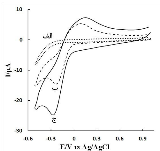
شکل ۲- ولتاموگرام‌های به‌دست‌آمده (الف) در غیاب و (ب و ج) به ترتیب در سطح الکتروود خمیر کربن و الکتروود خمیر گرافن در حضور محلول ۱ mM اورانیل در محلول بوریک اسید ۰/۱ مولار با pH=۳، سرعت اسکن ۵۰ میلی ولت بر ثانیه
