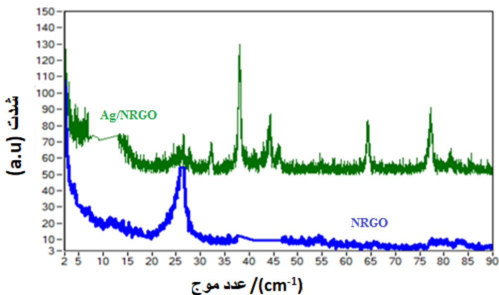
شکل ۱- نمودار XRD مربوط به NRGO و Ag / NRGO
