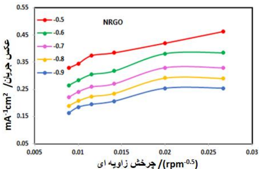
شکل ۵- نمودار لویج مربوط به ولتاژهای ۰/۵- تا ۰/۹- ولت برای کاتالیست NRGO شکل‌های ۵ و ۶، مربوط به پتانسیل‌های ۰/۵- تا ۰/۹- می باشد، این شکل‌ها از شکل‌های ۳ و ۴ استخراج شده است که با استفاده از شیب آنها می توان تعداد الکترون‌های مبادله شده را محاسبه کرد.
