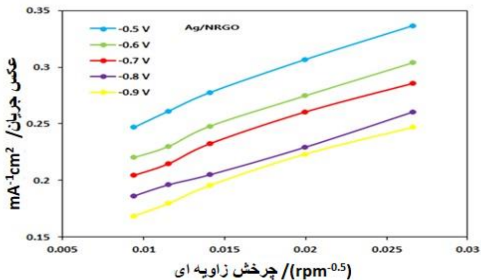
شکل ۵- نمودار لویج مربوط به ولتاژهای ۰/۵- تا ۰/۹- ولت برای کاتالیست NRGO شکل‌های ۵ و ۶، مربوط به پتانسیل‌های ۰/۵- تا ۰/۹- می باشد، این شکل‌ها از شکل‌های ۳ و ۴ استخراج شده است که با استفاده از شیب آنها می توان تعداد الکترون‌های مبادله شده را محاسبه کرد.
