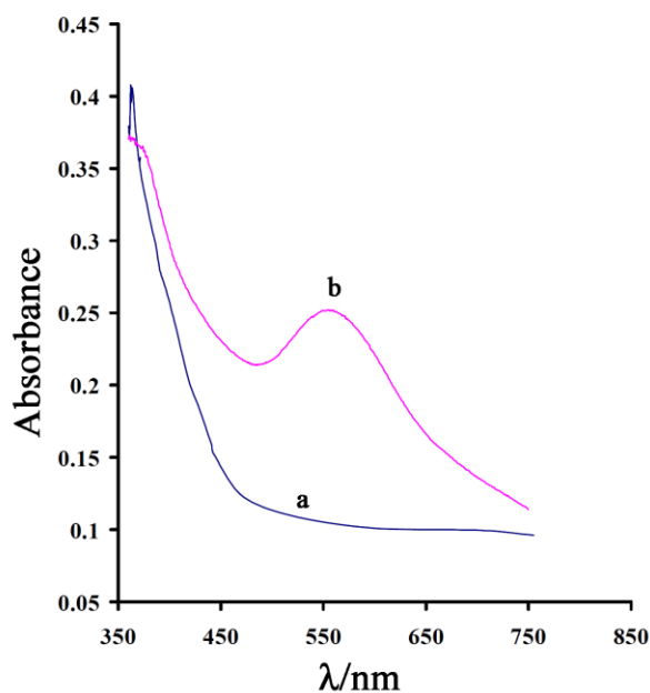
شکل (۱) طیف جذبی مرئی-فرابنفش نمک طلا (a) و نانوذرات طلا (b)
