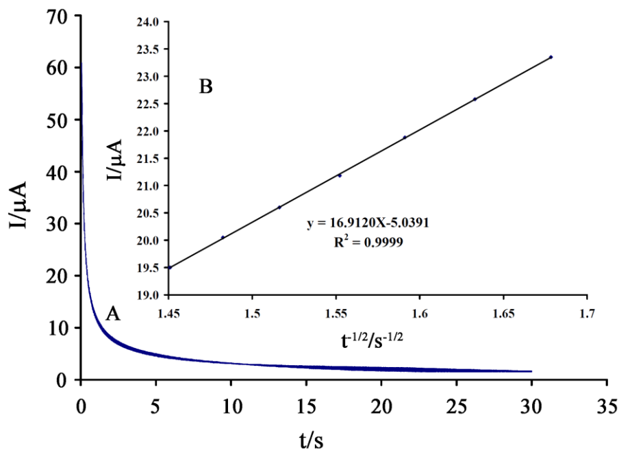
شکل ۷- کروئوآمپروگرام ۵۰۰ میکرومولار متیل دپا در سطح الکتروود اصلاح شده با مایع یونی و نانوذره طلا (A)، منحنی کاترل مستخرج شده از کروئوآمپروگرام (B).
