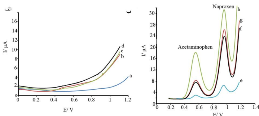
شکل ۳-۶ - ولتاموگرام (الف) محلول بافر در سطح الکتروود خمیر کربن (a) و الکتروود خمیر کربن اصلاح شده با نانوذرات NiCuFe_2O_4 (b)، الکتروود CNPE (c)، الکتروود اصلاح شده با MWCNTs/NiCuFe_2O_4/CPE (d) - ولتاموگرام (ب) مانند ولتاموگرام الف در حضور 300 \mu M میکرومولار ناپروکسن و 600 \mu M میکرومولار استامینوفن
