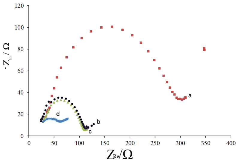
شکل ۳-۷ - امپدانس الکتروکود خیمیر کربن (a) ، الکتروکود CNPE (b) ، الکتروکود NiCuFe 2 O 4 /CPE (c) ، الکتروکود (d) MWCNTs/NiCuFe 2 O 4 /CPE.
