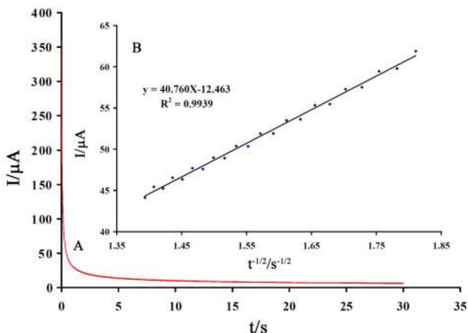
شکل ۶- کروئوآمپروگرام به دست آمده برای الکتروود خمیر کربن اصلاح شده با نانوذره فریت کبالت و مایع یونی در حضور غلظت ۵۰۰ میکرومولار بنزرازید در محلول بافر فسفات ۷/۰ pH (B) منحنی‌های کاترل به دست آمده از کروئوآمپروگرام
