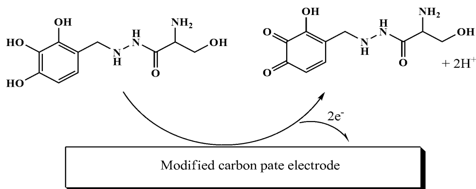
شکل ۲- مکانیزم اکسایش بنزرازید در سطح الکترواد [۱۸]
