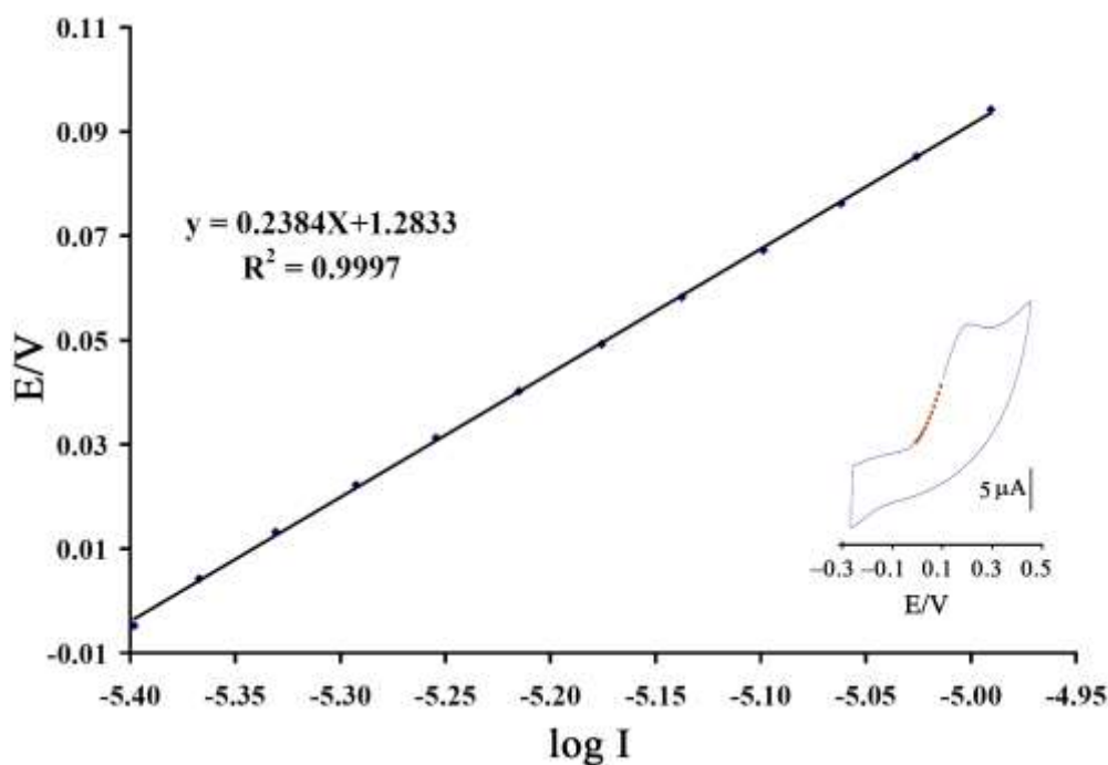
شکل ۵- نمودار تافل برای الکتروود اصلاح شده با نانوذره فریت کبالت و مایع یونی در حضور بنزآزید بافر فسفات ۱/۰ مولار pH=۷/۰
