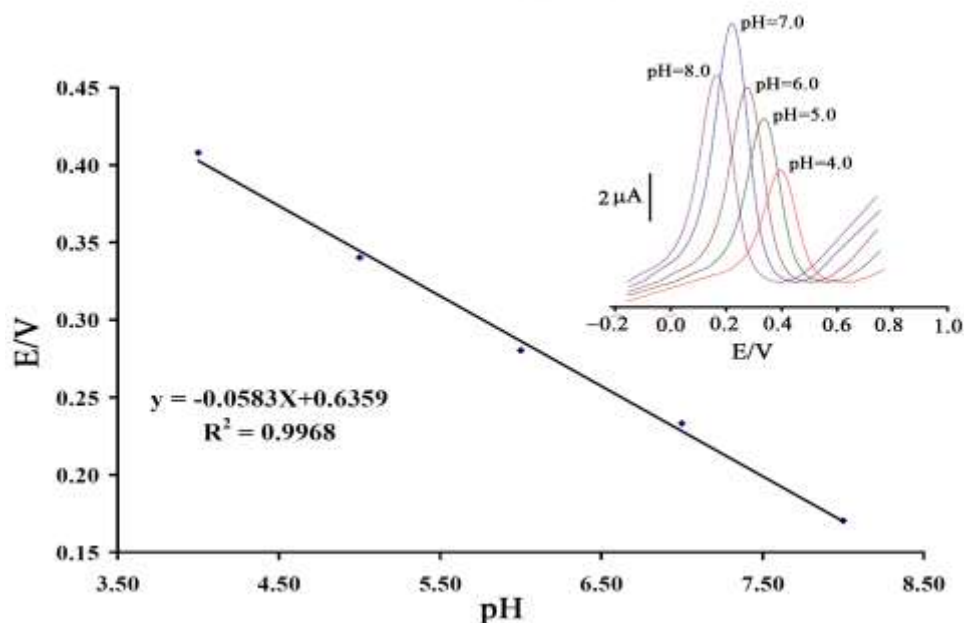
شکل ۳- منحنی تغییرات پتانسیل برحسب pH برای الکترواکسیداسیون ۷۵/۰ میکرومولار بنزرازید. شکل داخلی) ولتاموگرام موج مربعی ۷۵/۰ میکرومولار بنزرازید بر در pH بین ۴/۰ تا ۸/۰
