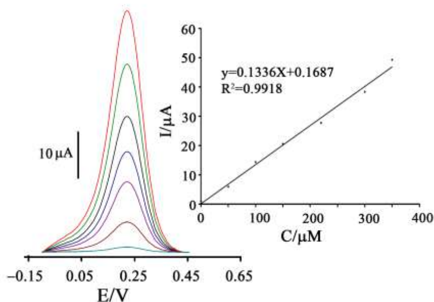
شکل ۷- ولتاموگرام‌های موج مربعی الکتروود اصلاح شده در حضور غلظت‌های ۰/۱، ۵۰/۰، ۱۰۰/۰، ۱۵۰/۰، ۲۲۰/۰، ۳۰۰/۰ و ۳۵۰/۰ میکرومولار بنزآزید و منحنی تغییرات شدت جریان آندی بر حسب تغییرات غلظت بنزآزید، pH=۷/۰.
