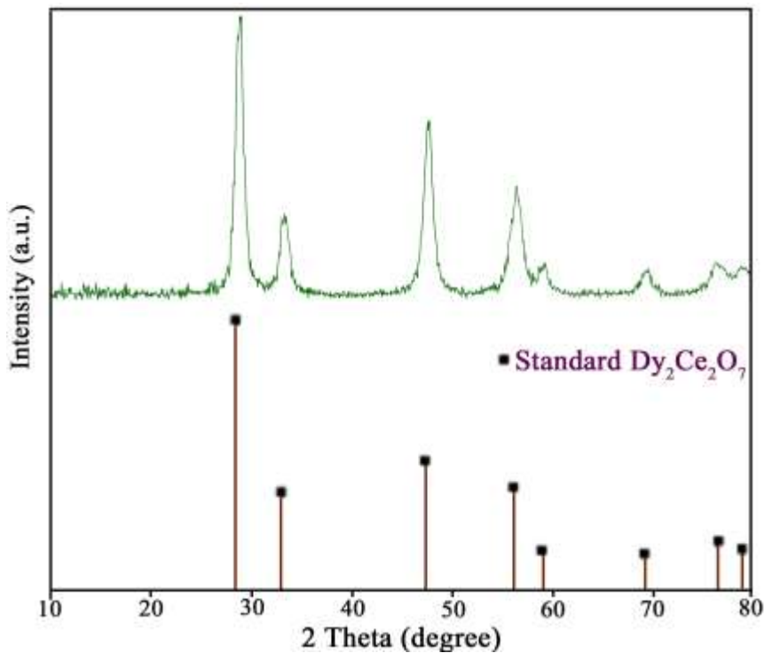
شکل ۱- الگوی XRD مربوط به نانوساختارهای Dy 2 Ce 2 O 7
