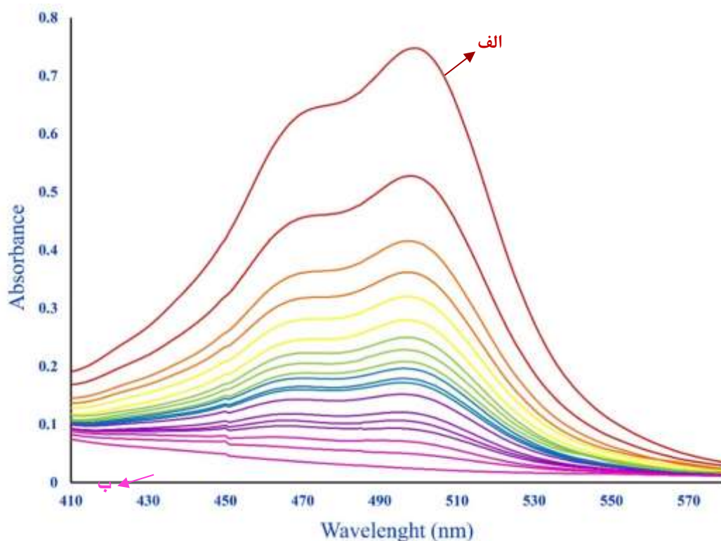
شکل ۱- تغییرات طیف UV-Vis در طی انجام واکنش اکسایش-افزایش [PtMe 2 (4,4'-Me 2 bpy)] (۳ mL) با غلظت 10^{-4} M و 3 \times 10^{-4} و [SnMe 2 (SCN) 2 ] با نسبت مولی ۱:۱ در حلال تولوئن در دمای اتاق، الف) [PtMe 2 (4,4'-Me 2 bpy)] خالص، ب) پس از گذشت ۹۰ دقیقه؛ حدفاصل ثبت ده طیف اول ۹۰ ثانیه است.
