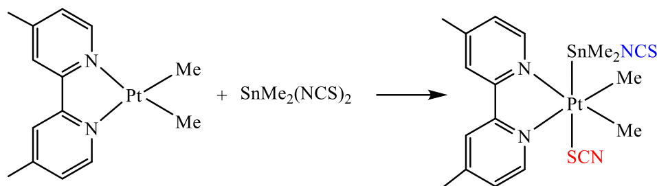
شماي ۱- روش تهیه کمپلکس (۳) trans-[PtMe_2(SnMe_2NCS)(SCN)(4,4'-Me_2bpy)]
