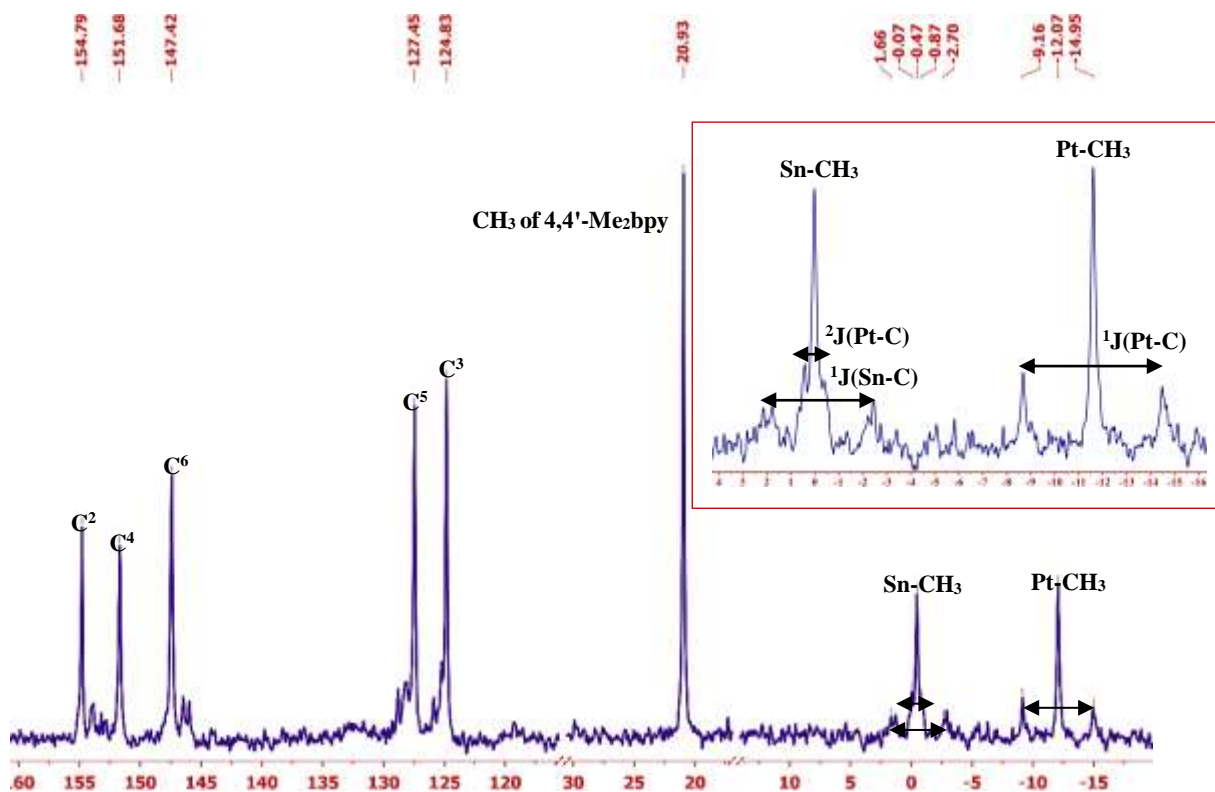
شکل ۳- طیف ^{13}\text{C} NMR کمپلکس (۳) trans\text{-}[\text{PtMe}_2(\text{SnMe}_2\text{NCS})(\text{SCN})(4,4'\text{-Me}_2\text{bpy})] در حلال \text{DMSO-}d_6 .
