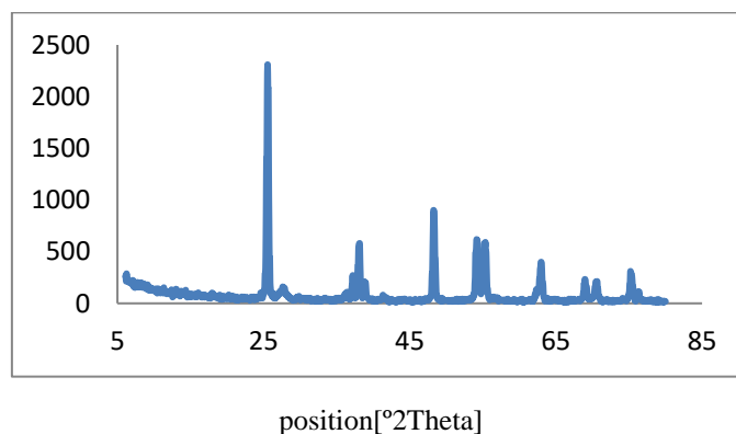
شکل ۴ الگوی پراش پرتو ایکس دی اکسید تیتانیوم روتایل
