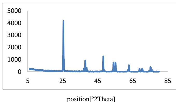
شکل ۳ الگوی پراش پرتو ایکس دی اکسید تیتانیوم آناتاز
