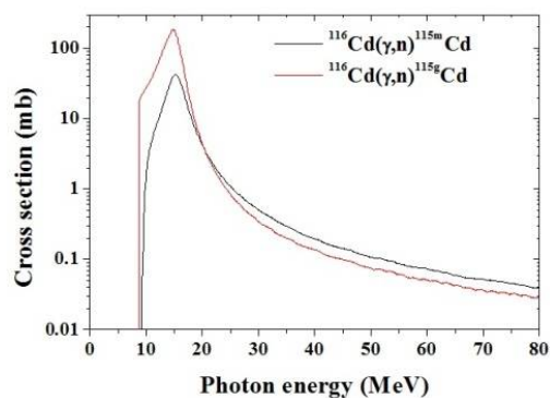
شکل ۴. سطح مقطع تولید هسته‌های ^{115m}\text{gCd} در واکنش ^{116}\text{Cd}(\gamma, n) .
