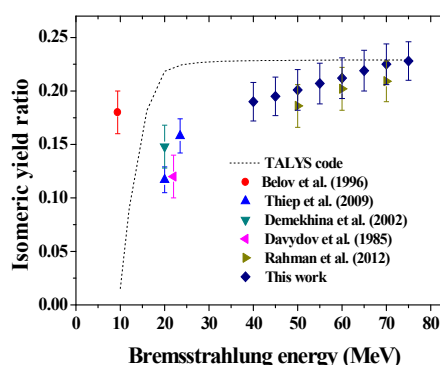
شکل ۵. وابستگی نسبت بهره ایزومری به انرژی فوتون‌های تابش ترمزی فرودی برای تولید جفت‌های ایزومری ^{115m}\text{gCd} .
