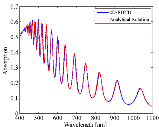
شکل ۳. تأثیر مدهای فابری پرو بر افزایش جذب درون سلول.
