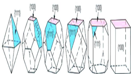
شکل 4. تغییرات ریخت شناسی در بلورهای fcc [30].
