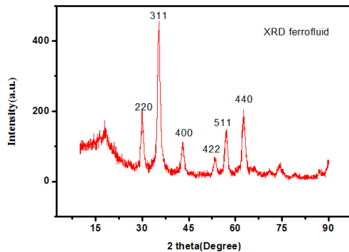
شکل 2 الگوی پراش اشعه ایکس فروسیال.
