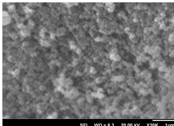
شکل (۲): عکس SEM نانوذرات \text{CaF}_2:\text{Ti}
