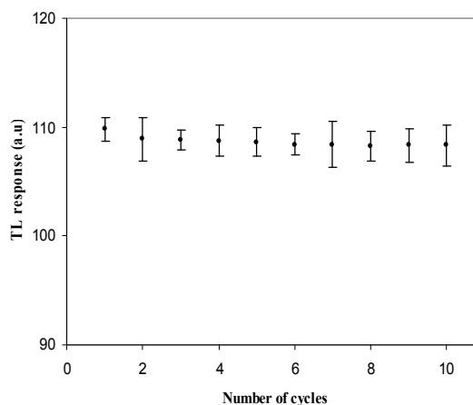
شکل (۷): تکرارپذیری نانوذرات \text{CaF}_2:\text{Ti} برای ده مرتبه پی‌در پی از گرمادهی، پرتودهی و قرائت
