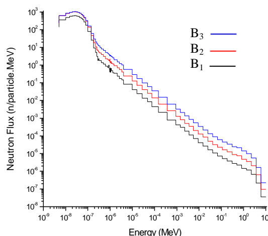
شکل ۴: طیف نوترون در ابتدای بیم تیوبها در حالت BOC.
