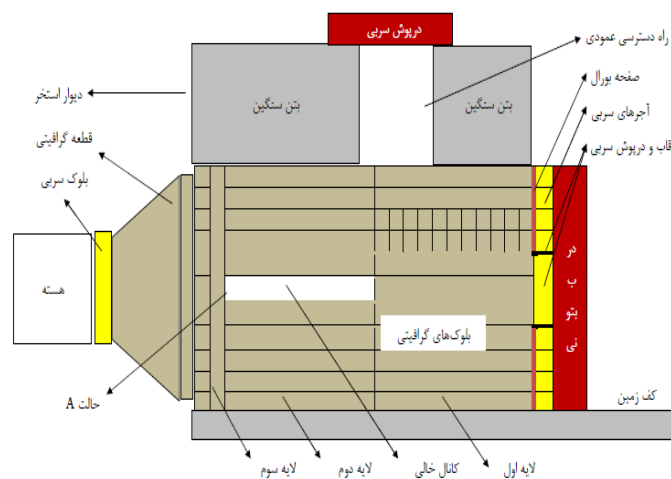
شکل (۱): ساختار ستون حرارتی راکتور تهران
