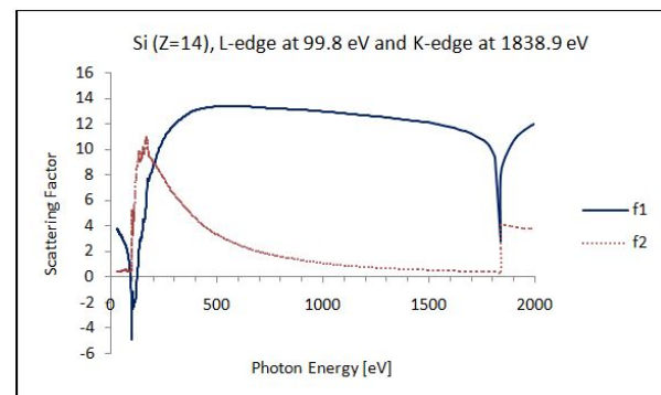
شکل (۳): تغییرات f_1 و f_2 در نزدیکی لبه‌های جذب K و L در Si
