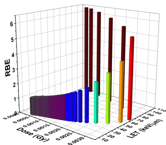
شکل (۱): تغییرات RBE برحسب دز فیزیکی و LET.
