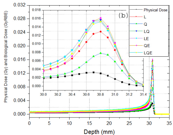
شکل ۵(ب): مقدار RBE و مقدار دز زیستی برای مدل‌های مختلف f(L) در تابش یون هلیوم با انرژی E=248 \text{ MeV} .
