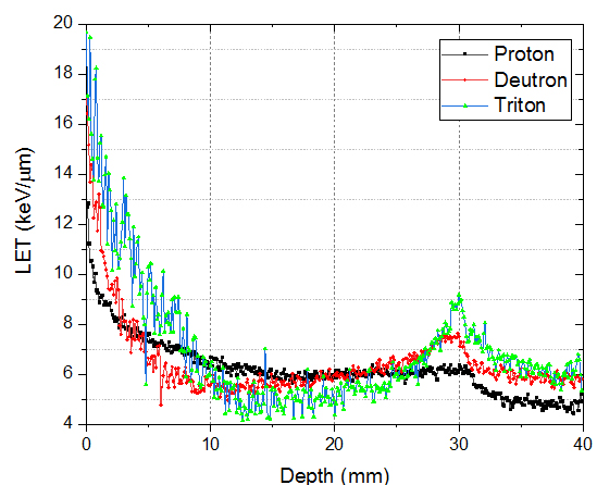
شکل (۶): مقدار LET مربوط به ذرات ثانویه با Z=1 حاصل از تابش یون هلیوم با انرژی E=248 MeV.
