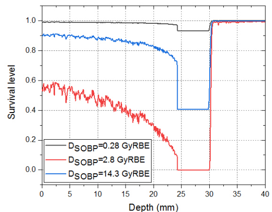
شکل (۱۰): سطح بقای سلولی در تابش دسته پرتو یون هلیوم. پارامتر D_{SOBP} مقدار دز زیستی در ناحیه SOBP را نشان می دهد.
