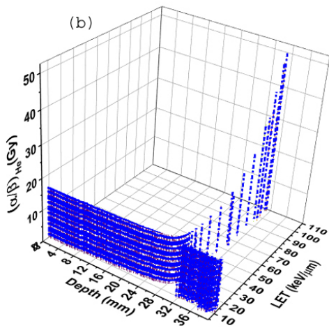
شکل ۵(a): مقدار (\alpha/\beta)_{He} بر حسب عمق در فانتوم با تابش یون هلیوم با انرژی E=248 \text{ MeV} . (b) تغییرات سه بعدی مقدار (\alpha/\beta)_{He} بر حسب LET و عمق در فانتوم.
