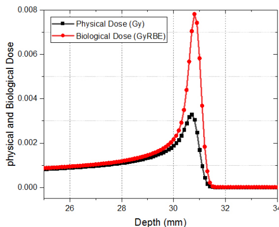
شکل (۲): مقایسه تفاوت قابل توجه دز زیستی نسبت به دز فیزیکی در تابش یون هلیوم با انرژی E=248 \text{ MeV} .
