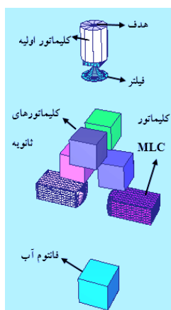
شکل (۱): نمایی سه بعدی از اجزاء شبیه‌سازی شده‌ی دستگاه واریان 2100 \text{ C/D} .
