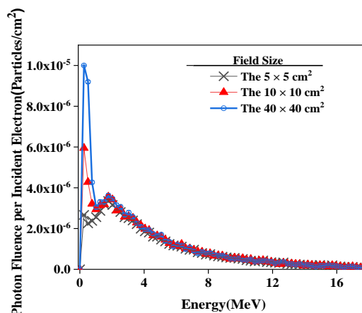
شکل (۷): طیف فوتون در عمق ۰,۵ cm درون فانتوم برای میدان‌های 5 \times 5 \text{ cm}^2 ، 10 \times 10 \text{ cm}^2 و 40 \times 40 \text{ cm}^2 .
