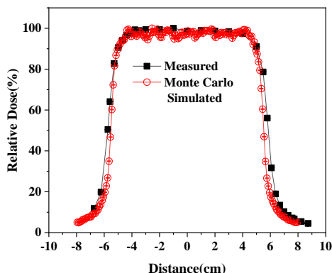
شکل (۳): مقایسه‌ی درصد دز پروفایل حاصل از اندازه‌گیری تجربی و
