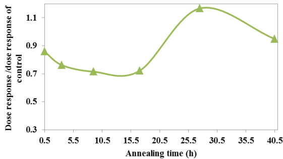
شکل (3): نسبت پاسخ نمونه‌ی TLD-400 به پاسخ نمونه‌ی کنترل به ازای مراحل مختلف گرمادهی و دریافت دز به میزان 1 Gy نشان داده شده است.
