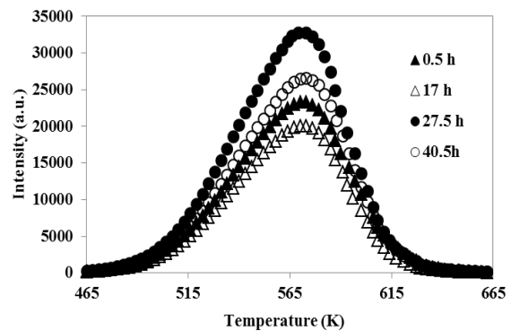
شکل (2): منحنی‌های تابش ترمولومینسانس دزیمتر TLD-400 بعد از دریافت دز 10 kGy و اعمال مراحل مختلف گرمادهی نشان داده شده است.
