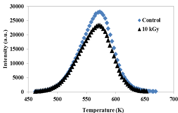
شکل (1): کاهش حساسیت دزیتر TLD-400 پس از دریافت دز به میزان 10\text{ kGy} ، اعمال فرآیند گرمادهی استاندارد و دریافت مجدد دز به میزان 1\text{ Gy} ، در مقایسه با دزیتر کنترل نشان داده شده است.
