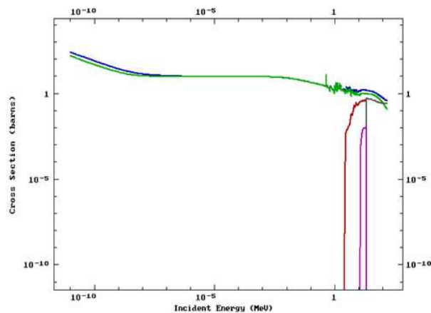
شکل (۲): سطح مقطع برهم کنش نوترون با هدف نیتروژن بر حسب انرژی.
