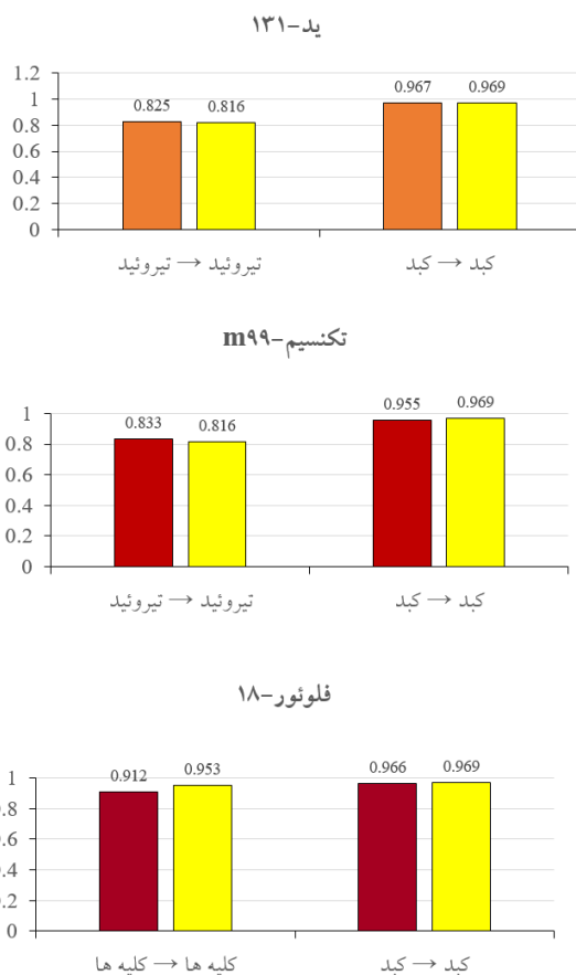
شکل (۷): نسبت مقادیر S در دز خود جذبی برای اندام چشمه تیروئید، کلیه‌ها و کبد در مقایسه با نسبت جرم آن‌ها.
