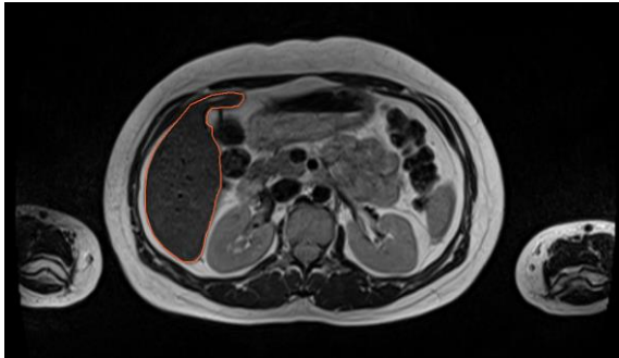
شکل (۱): تصویر مقطعی از بدن فرد داوطلب که توسط دستگاه ام‌آرآی گرفته شده است. مرزبندی اندام کبد در این تصویر مشاهده می‌شود.
