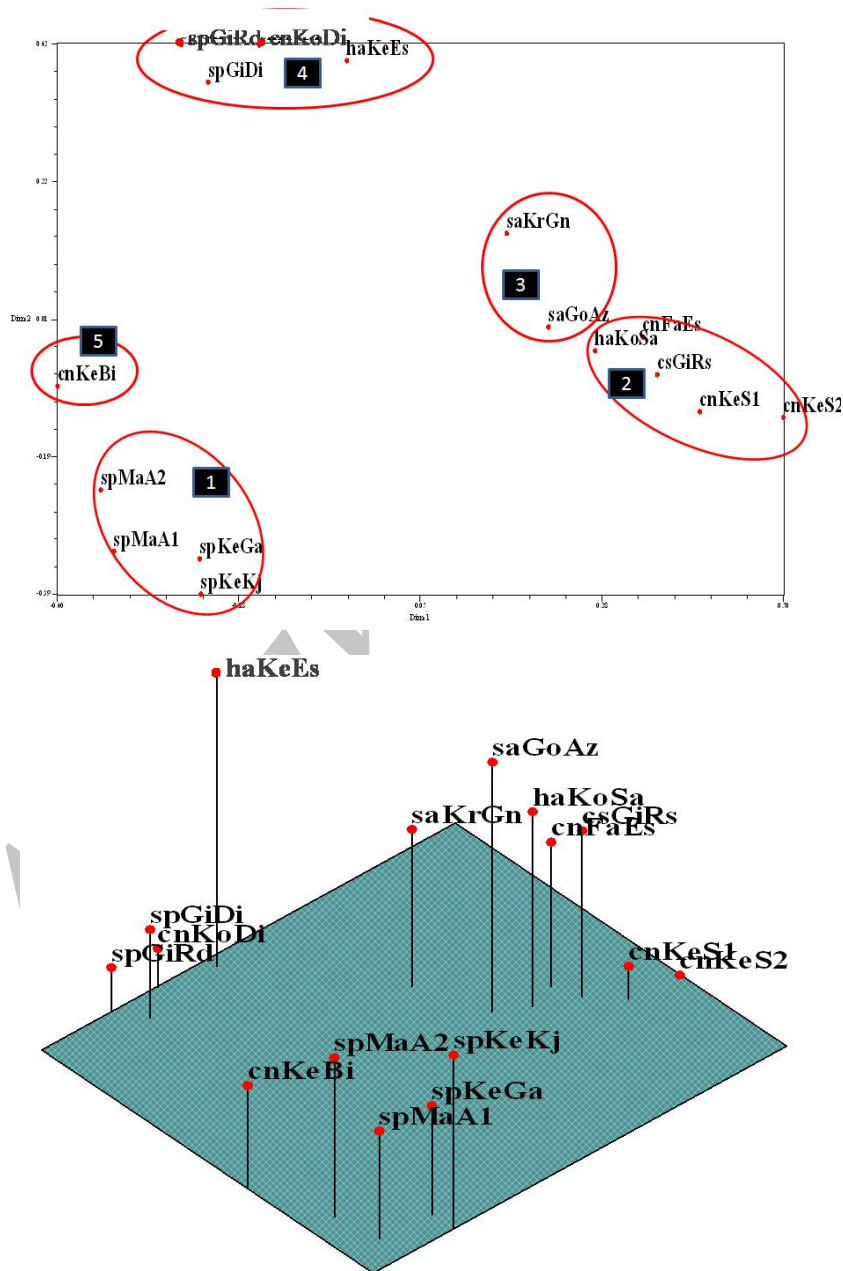
شکل ۴- نمودار دو بعدی (بالا) و سه بعدی (پایین) تجزیه به مولفه های اصلی بر اساس فراوانی داده های نشانگر ISSR
