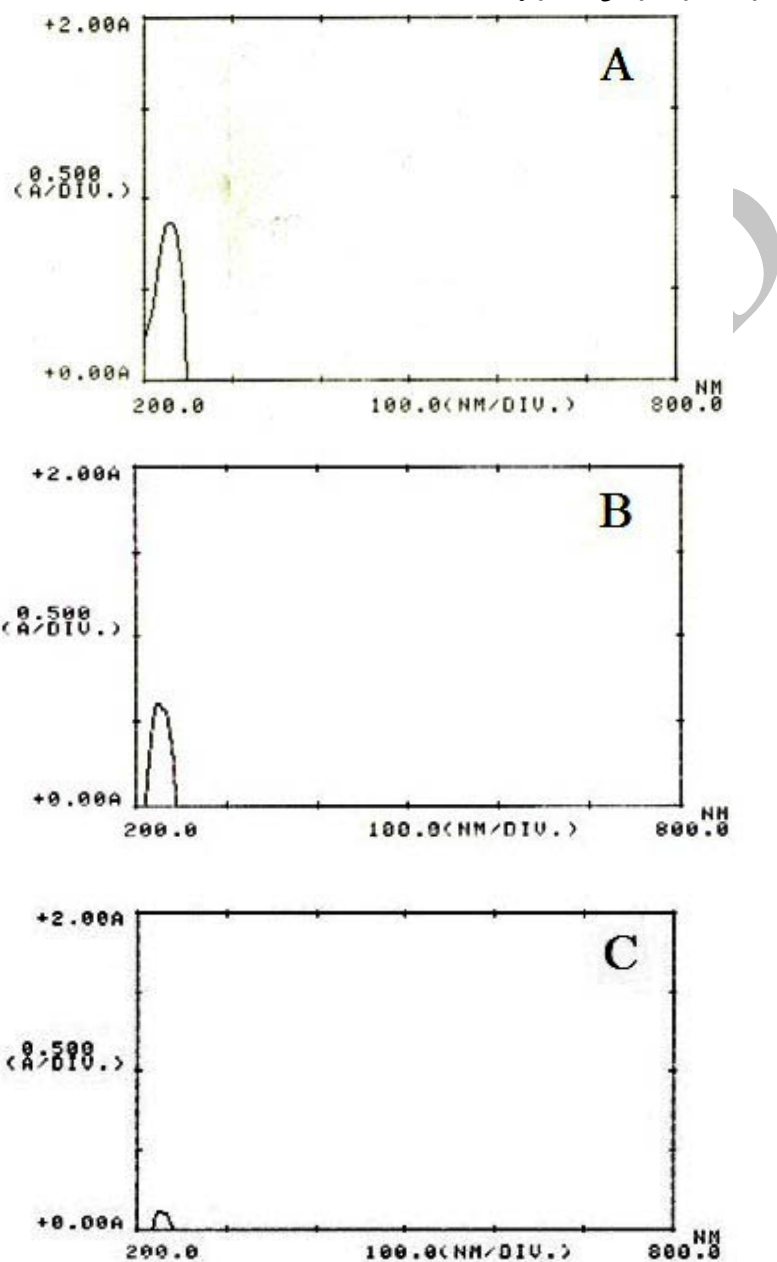
شکل ۲- جذب UV تیوفن در طول موج ۲۳۰ نانومتر توسط سلول‌های فعال بدون رشد باکتری پس از ۱۵ ساعت گرماگذاری در دمای ۳۰ درجه سانتی‌گراد: (A) نمونه کنترل بدون باکتری با رقت ۱/۵۰ (B) نمونه حاوی باکتری با رقت ۱/۲ (C) نمونه حاوی باکتری با رقت ۱/۱۰. (محور افقی: طول موج بر حسب نانومتر، محور عمودی: میزان جذب UV)
