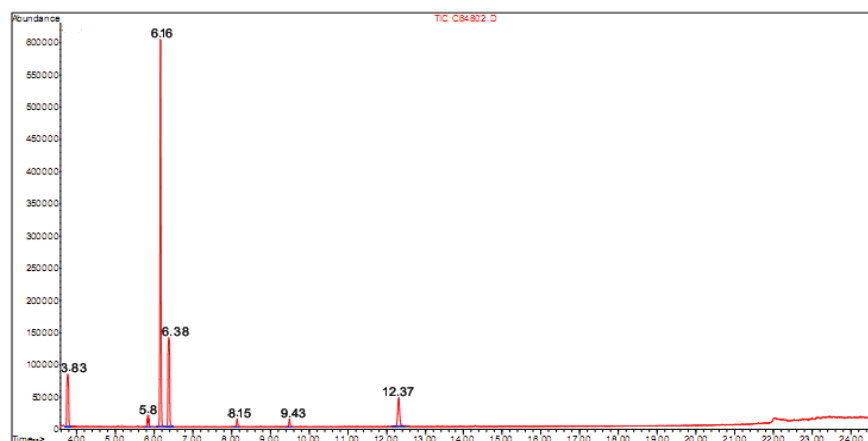
شکل ۴- طیف GC، مربوط به رسوب حاصل از استخراج DNA
