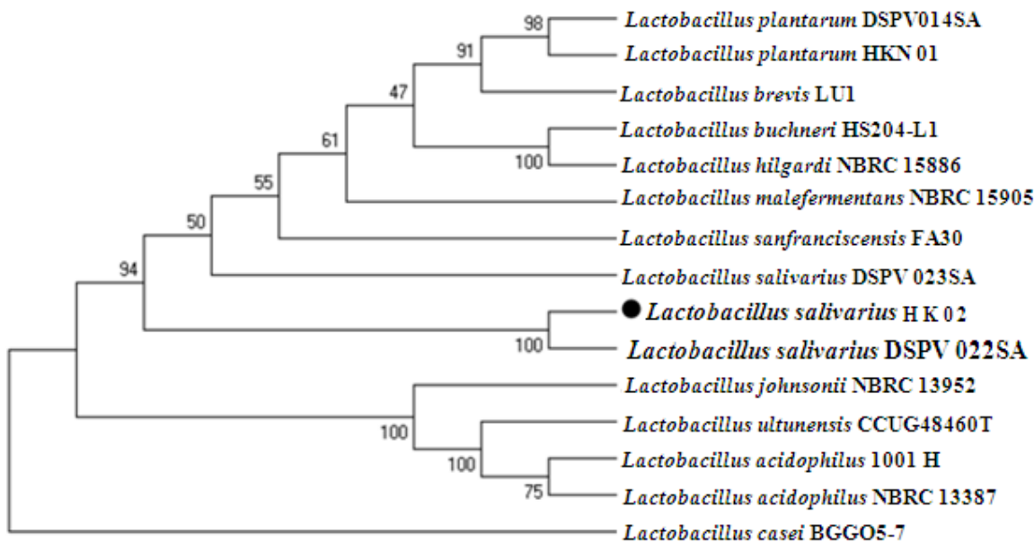
شکل ۲- فیلوژنتیک دندروگرام حاصل از آنالیز توالی rRNA ۱۶S. ارتباط سویه NK02 با دیگر لاکتوباسیلوسها نشان داده شده است.
