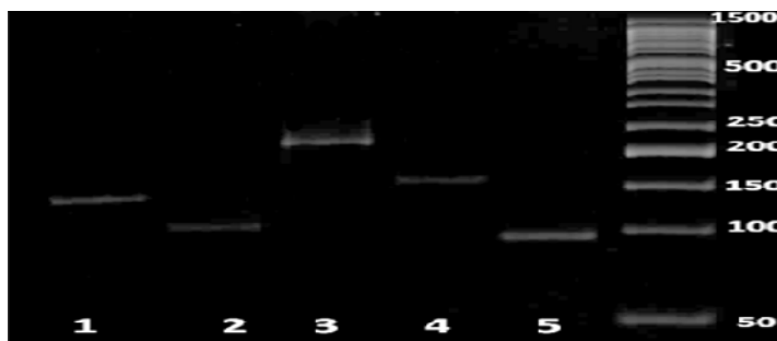
شکل ۲- قطعات جهش یافته برای تولید جهش‌های Y45W بر روی ژل آکریل آمید ۸ درصد: ستون‌های ۲ و ۴ به ترتیب قطعات 99bp و 169bp (به ترتیب حاصل از تکثیر پرایمرهای R, fI, tI, F)، ستون ۳ نشان دهنده قطعه 243bp جهش یافته Y45W حاصل از تکثیر قطعات ستون‌های ۲ و ۴ به عنوان template است. ستون‌های ۱ و ۵ مربوط به تکثیر قطعات با جهش‌های دیگر است.
