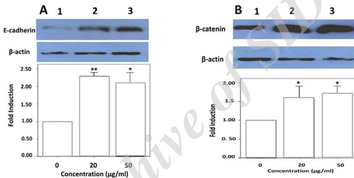
شکل ۳- بررسی تأثیر غلظت‌های ۲۰ و ۵۰ میکروگرم در میلی لیتر عصاره دانه انار بر مقدار سلولی پروتئین E-cadherin (A) و \beta -catenin (B) در سلول‌های PC-3 با استفاده از روش وسترن بلاتینگ. نتایج، میانگین حاصل از سه آزمایش مستقل می‌باشد (*: p < 0.05 و **: p < 0.01 ).
