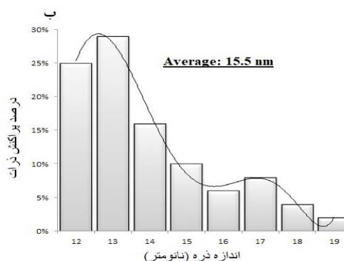
شکل ۷- (الف) تصویر SEM حاصل از نانو سولفید کادمیوم سنتز شده توسط سوپرنانانت کشتی P. pseudoalcaligenes Cd11 و (ب) هیستوگرام مربوط به دامنه پراکنش اندازه نانو سولفید کادمیوم سنتز شده.
