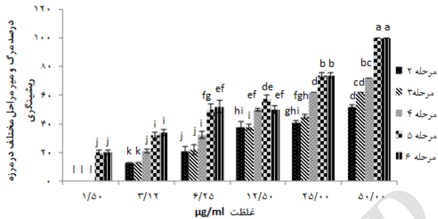
شکل ۱- مقایسه مربوط به اثرات غلظت های مختلف اسانس گیاه S. rechingeri بر مراحل مختلف لاروی بارناکل و مقایسه مراحل ناپلیوسی با یکدیگر. آنتنکها نشانهی انحراف معیار و حروف غیرمشابه نشان دهندهی تفاوت معنی دار بین غلظت های متفاوت اسانس می باشد.
