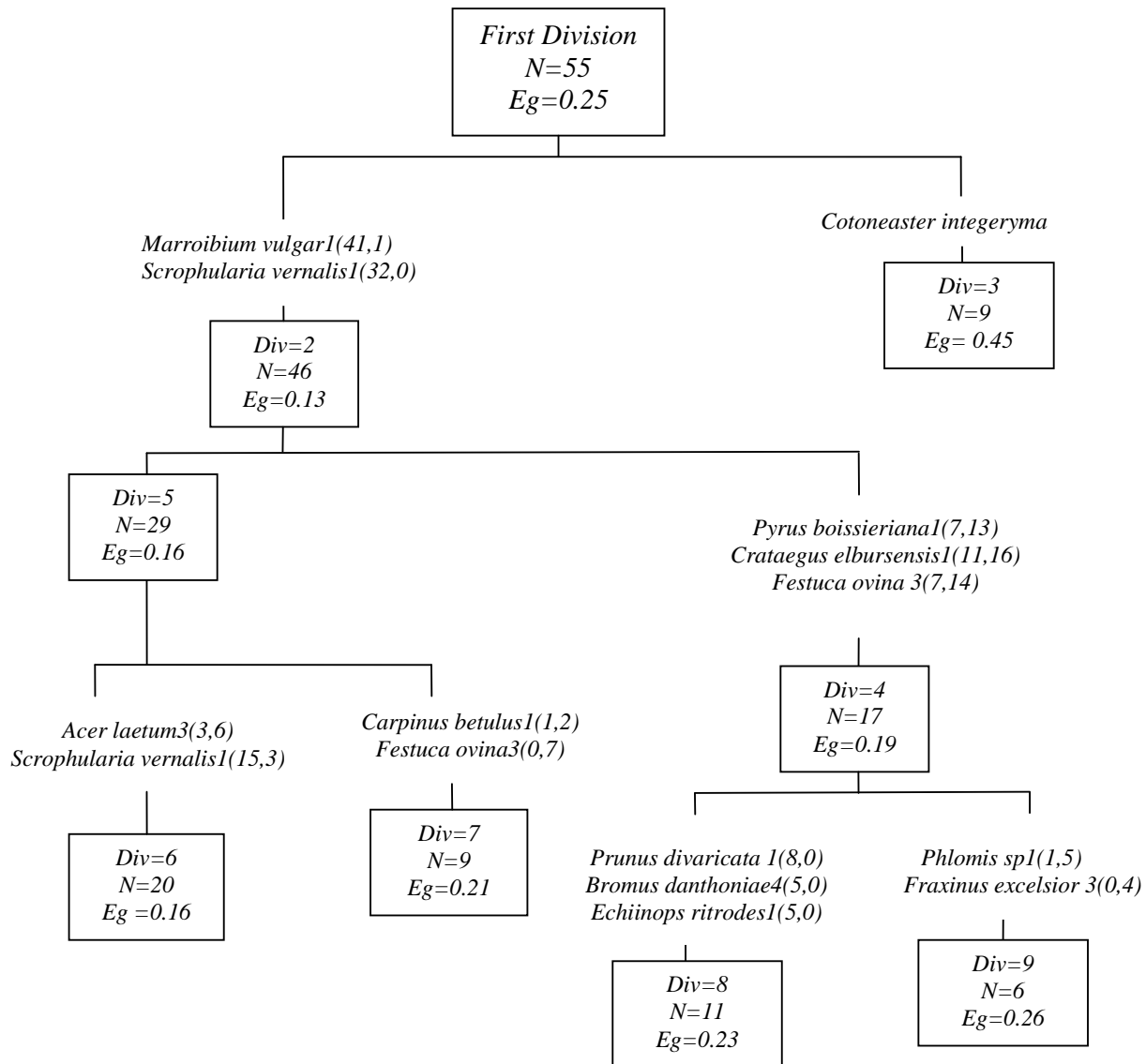
شکل ۲- طبقه‌بندی داده‌های پوشش گیاهی جنگل‌های جوزک- درکش با بهره‌گیری از تجزیه TWINSpan
